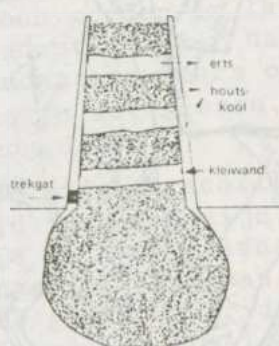
Een stoven voor het stoken, gereed met wisselend lagen houtskool en erts, ten dele ingegraven.
