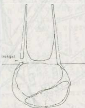
Oven bij het einde van de bewerking; het onderste deel van de oven is gevuld met slakken en ijzer.
