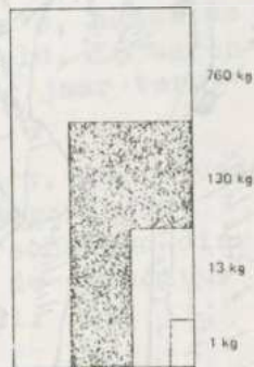
Bereiding van moerasijzererts. Om 1 kg bruikbaar ijzer te bereiden uit 13 kg moerasijzererts, werd 130 kg houtskool (760 kg rekenhout) gebruikt.
